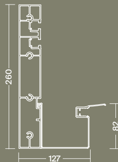
Gutter Gouttière
