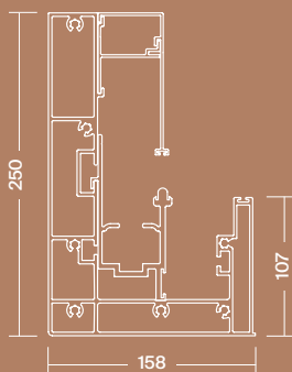
Gutter Gouttière
