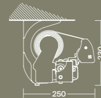
Ceiling installation 0° - 90° Installation au plafond 0° - 90°
