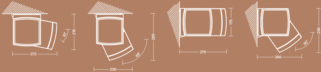
Instalación a techo 10° Instalação no teto 10°
