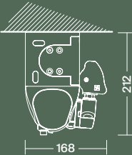
Ceiling installation 0° - 90° Installation au plafond 0° - 90°
