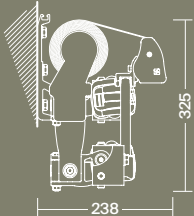
Wall installation with crossed arms Installation murale avec bras croisés
