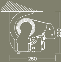
Ceiling installation 0° - 90° Installation au plafond 0° - 90°
