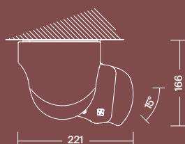
Ceiling installation 15° Installation au plafond 15°
