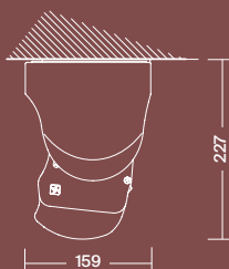
Ceiling installation 90° Installation au plafond 90°
