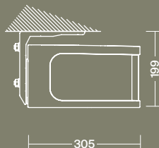
Ceiling installation Installation au plafond
