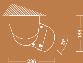
Ceiling installation 15° Installation au plafond 15°
