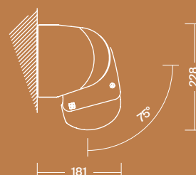
Instalación a pared 75° Instalação na parede 75°
