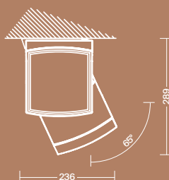
Instalación a techo 65° Instalação no teto 65°
