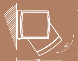
Instalación a pared 55° Instalação na parede 55°
