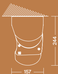
Instalación a techo 90° Instalação no teto 90°
