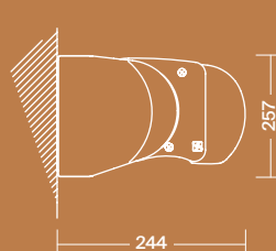
Instalación a pared Instalação na parede
