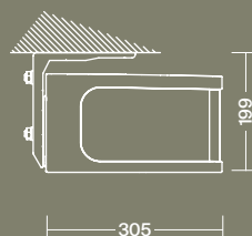
Instalación a techo Instalação no teto
