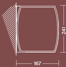
Instalación a pared con terminal cofre Instalação na parede com terminal de cofre
