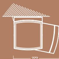
Instalación a techo 10° Instalação no teto 10°
