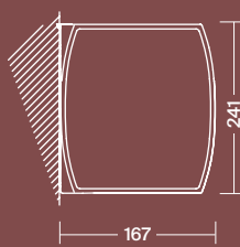
Instalación a pared con terminal cofre Instalação na parede com terminal de cofre
