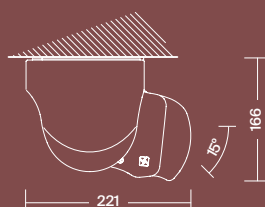
Instalación a techo 15° Instalação no teto 15°
