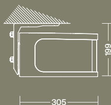
Instalación a techo Instalação no teto
